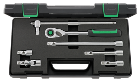
96034010 Satz Betätigungswerkzeuge
